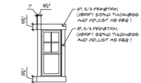
WINDOW TRIM DETAIL SCALE: 3/8" = 1'-0"
